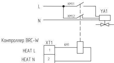
Подключение электромагнитного прибора двух-/трехходового вентиля без возвратной пружины:
