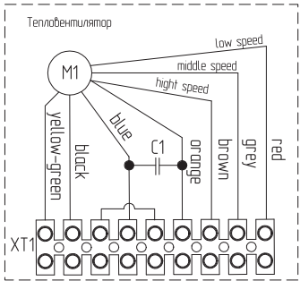
Внутренняя схема клеммной коробки тепловентилятора.
