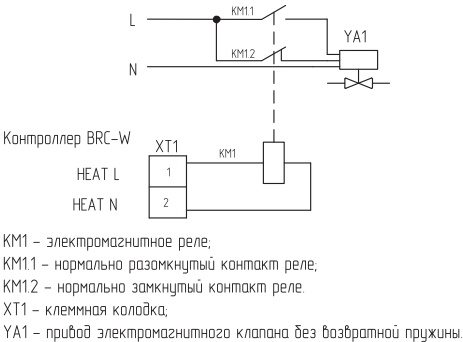
Подключение электромагнитного привода двух-/трехходового вентиля без возвратной пружины:
